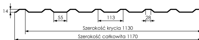
Schemat techniczny
