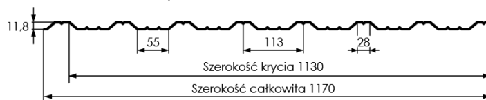
Schemat techniczny
