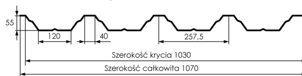
Schemat techniczny
