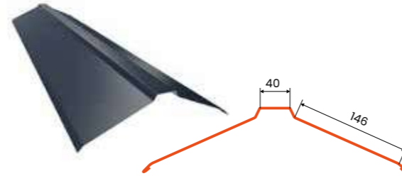
gąsior trapez PHR
