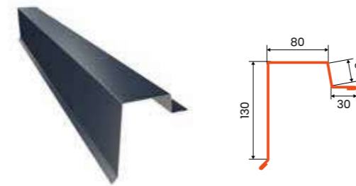
wiatrownica PHR
