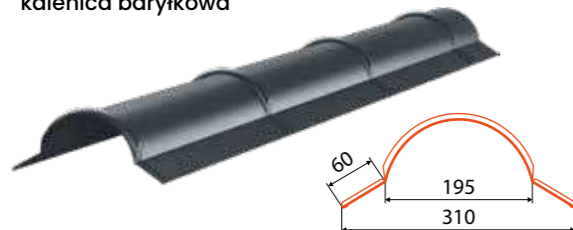
kalenica baryłkowa
